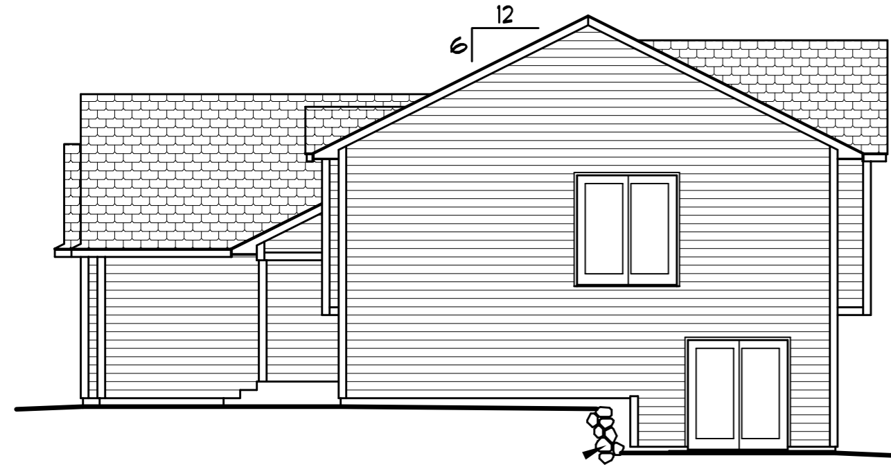
RIGHT ELEVATION
