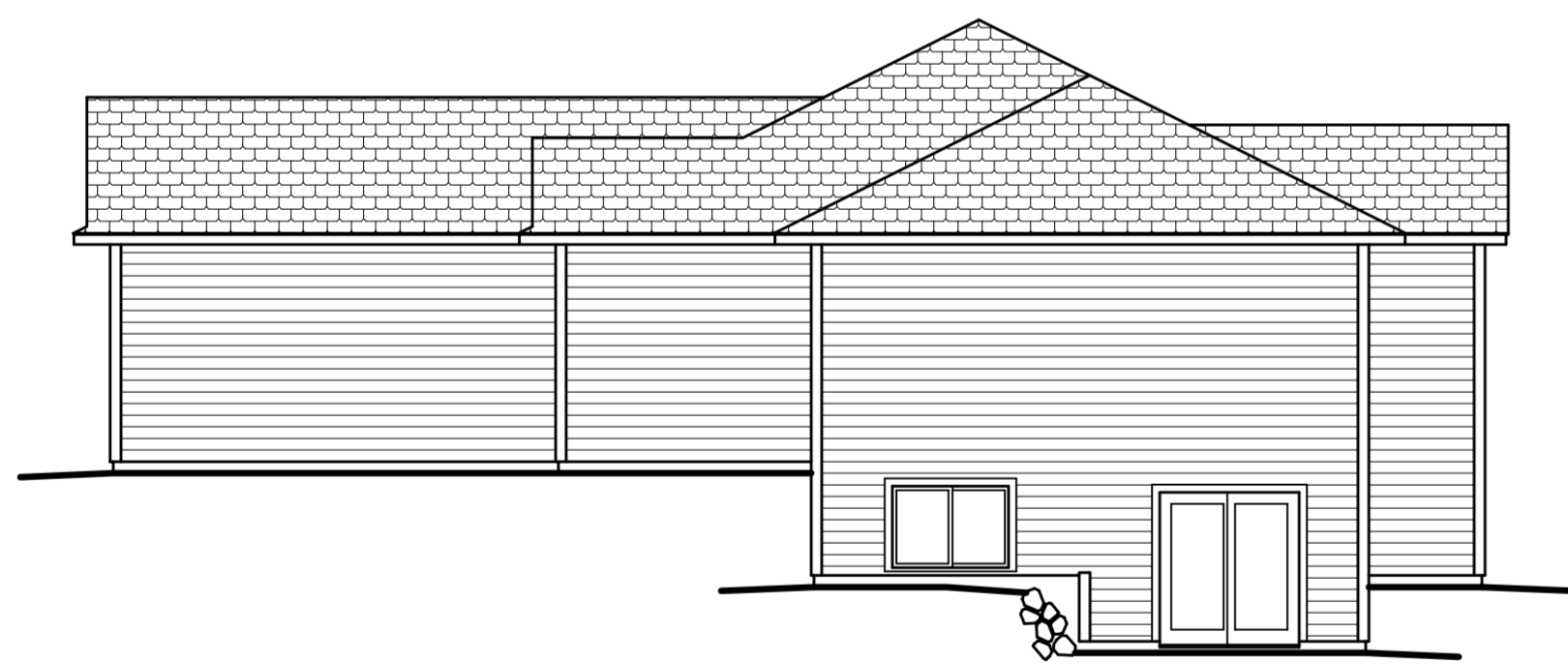
RIGHT ELEVATION
